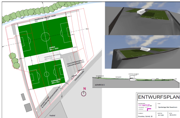
Entwurfsplan der neuen Sportplatzanlage in der Eisenstädterstraße
